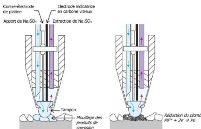
Fig. 2: Vue en coupe du principe de fonctionnement du Pleco : création de la cellule électrolytique (à gauche) et réduction des produits de corrosion (droite)
